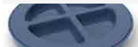
CFC2H
