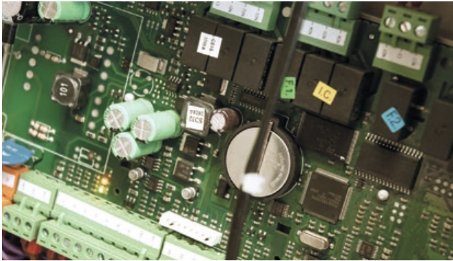
PID Temperaturregler Platine
