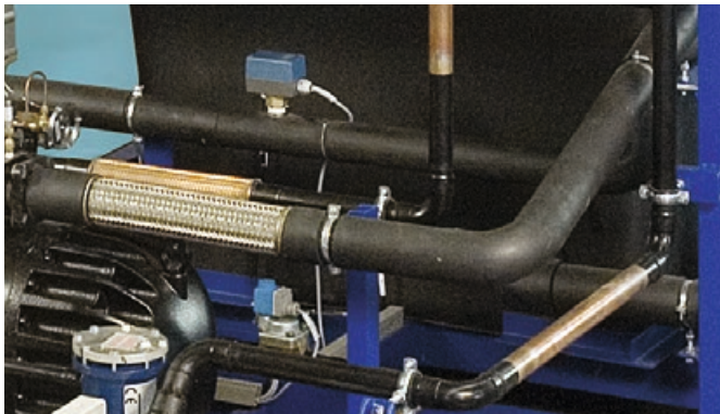
Baureihe RKH-R mit Radialverflüssiger zum Luftkanalanschluss
